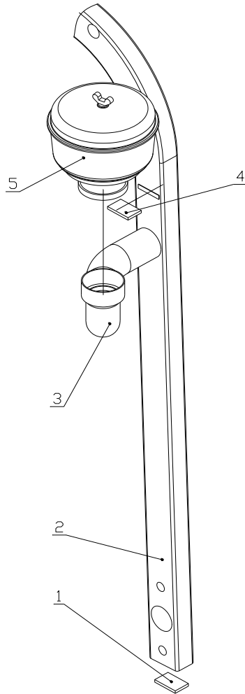
图 56 高位进气系统 Fig. 56 High Air intake system
