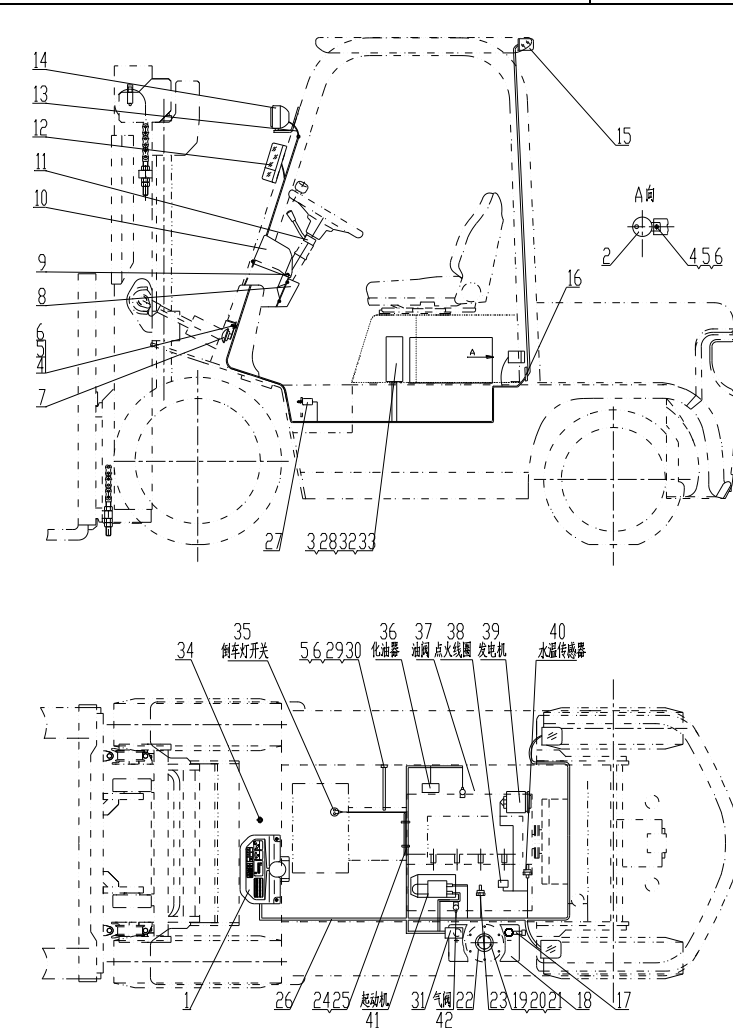
图 10-1 电气系统 Fig.10-1 Electrical system
