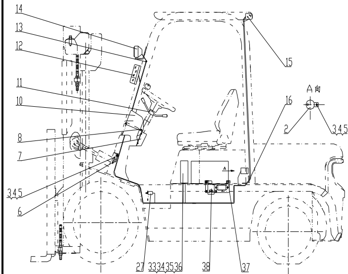
图 1-2 电气系统 Fig.1-2 Electrical system
