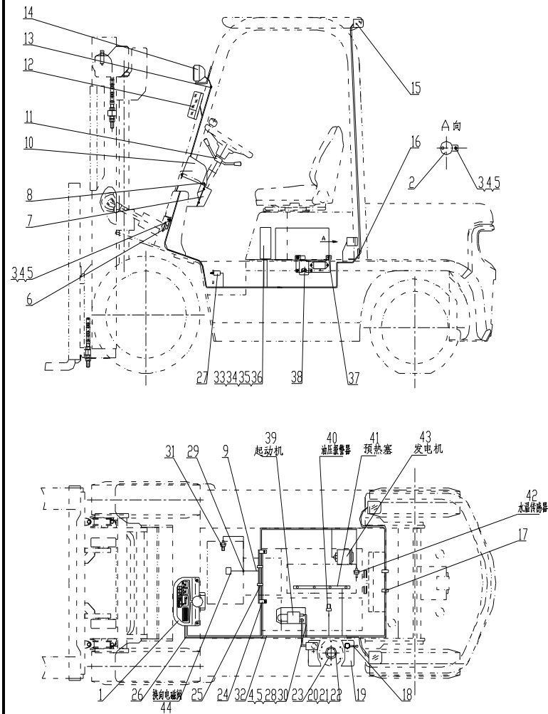
图 2-2 电气系统 Fig.2-2 Electrical system
