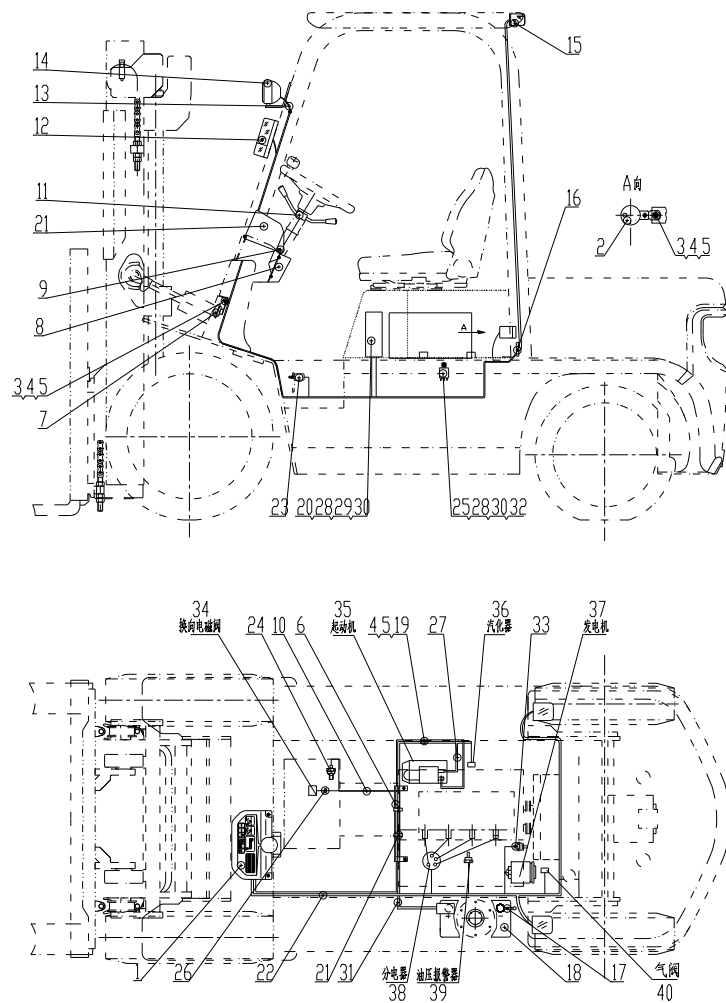
图9 电气系统 Fig.9 Electrical system
