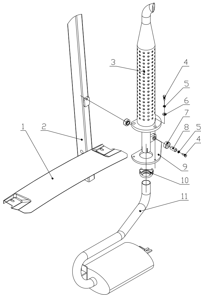
图 61 高位排气系统 Fig.61 High Exhaust system
