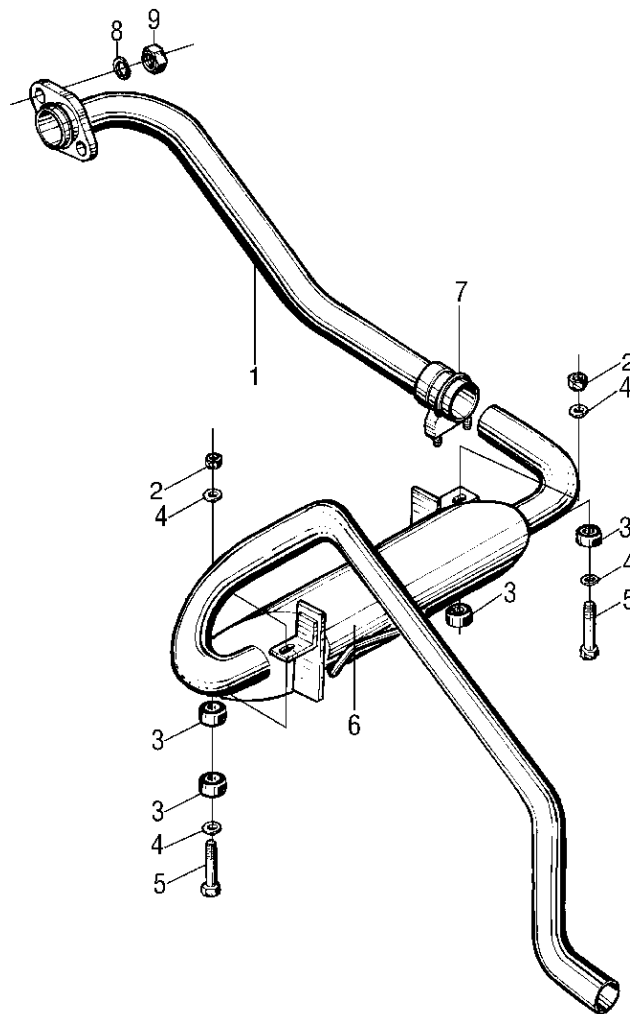
图 47 排气系统 Fig.47 Exhaust system
