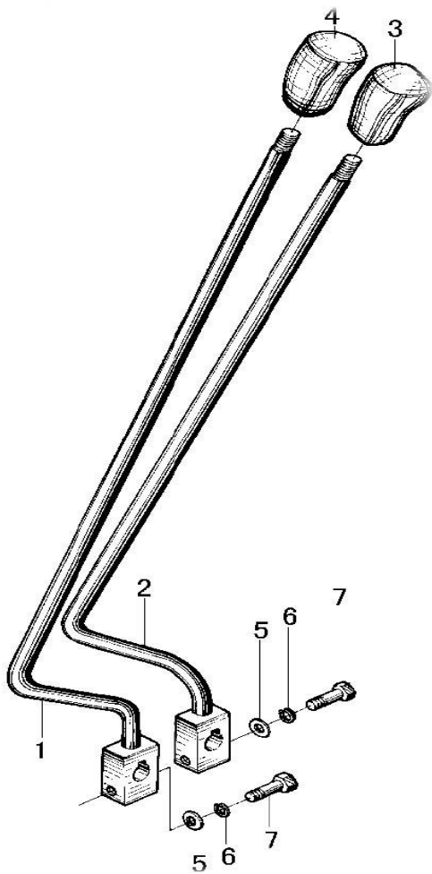
图 13 换档操纵总成 Fig. 13 Change over control assy
