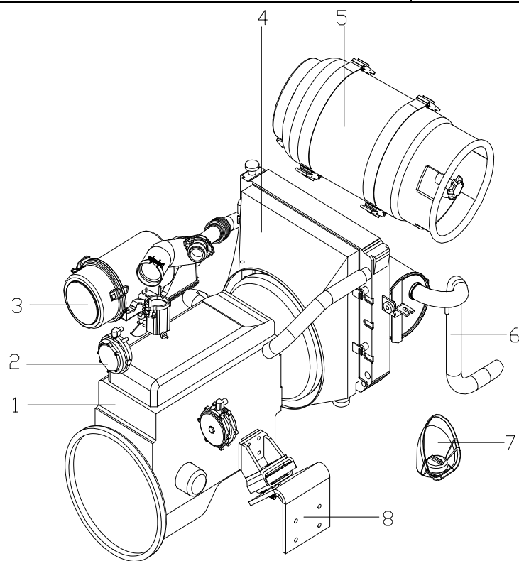
图 41 动力系统 Fig. 41 Power system
