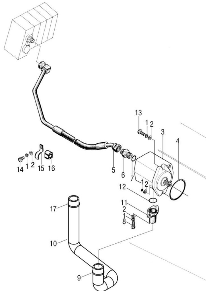
图 2 油泵总成 Fig.2 Pump assy
