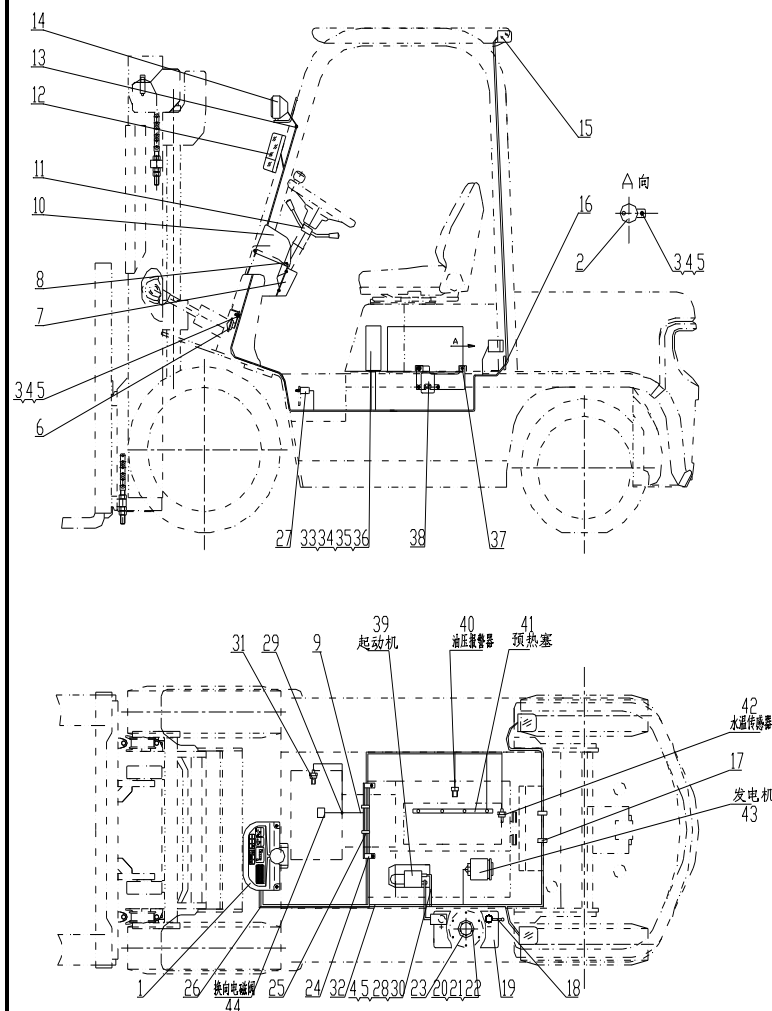
图 8 电气系统 Fig. 8 Electrical system
