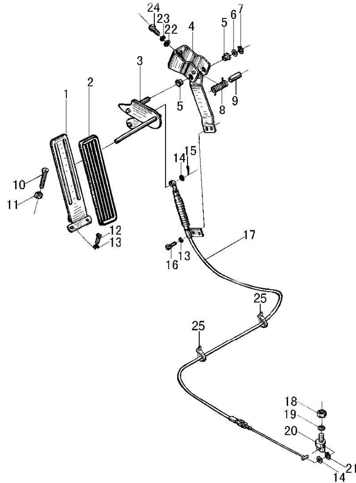
图 12 油门操纵总成 Fig. 12 Throttle control assy
