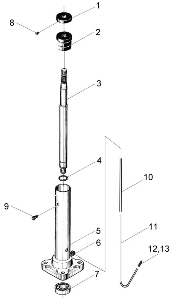
图 6 转向管装置 Fig. 6 Steering pipe device
