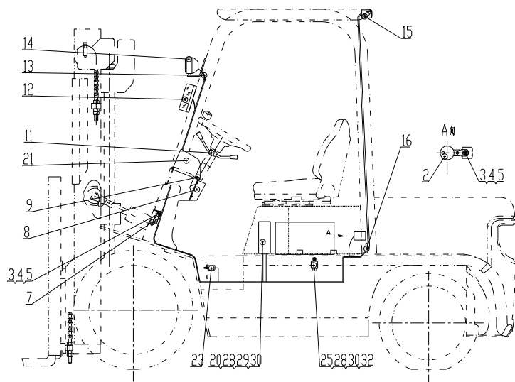
图9 电气系统 Fig.9 Electrical system
