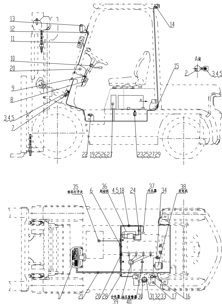
图 6-1 电气系统 Fig.6-1 Electrical system
