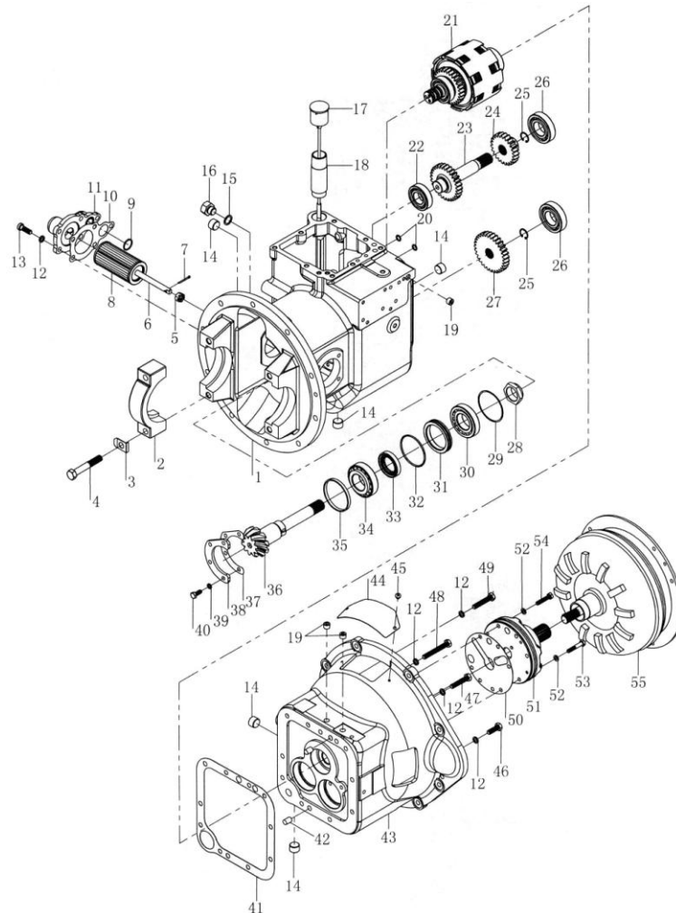
图 18 变速箱（液力式）绍兴 SHAOXIN Fig. 18 Transmission(tor-con type)
