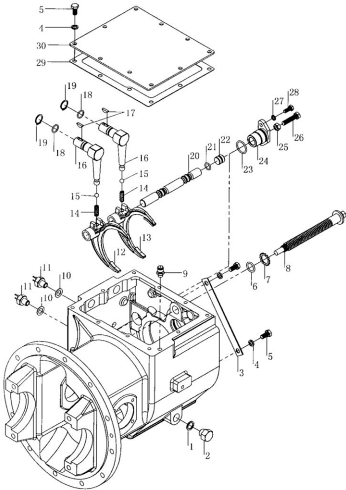
图 16 变速器(机械式 其 1) 绍兴 ShaoXin Fig.16 Transmission(clutch type part-1)
