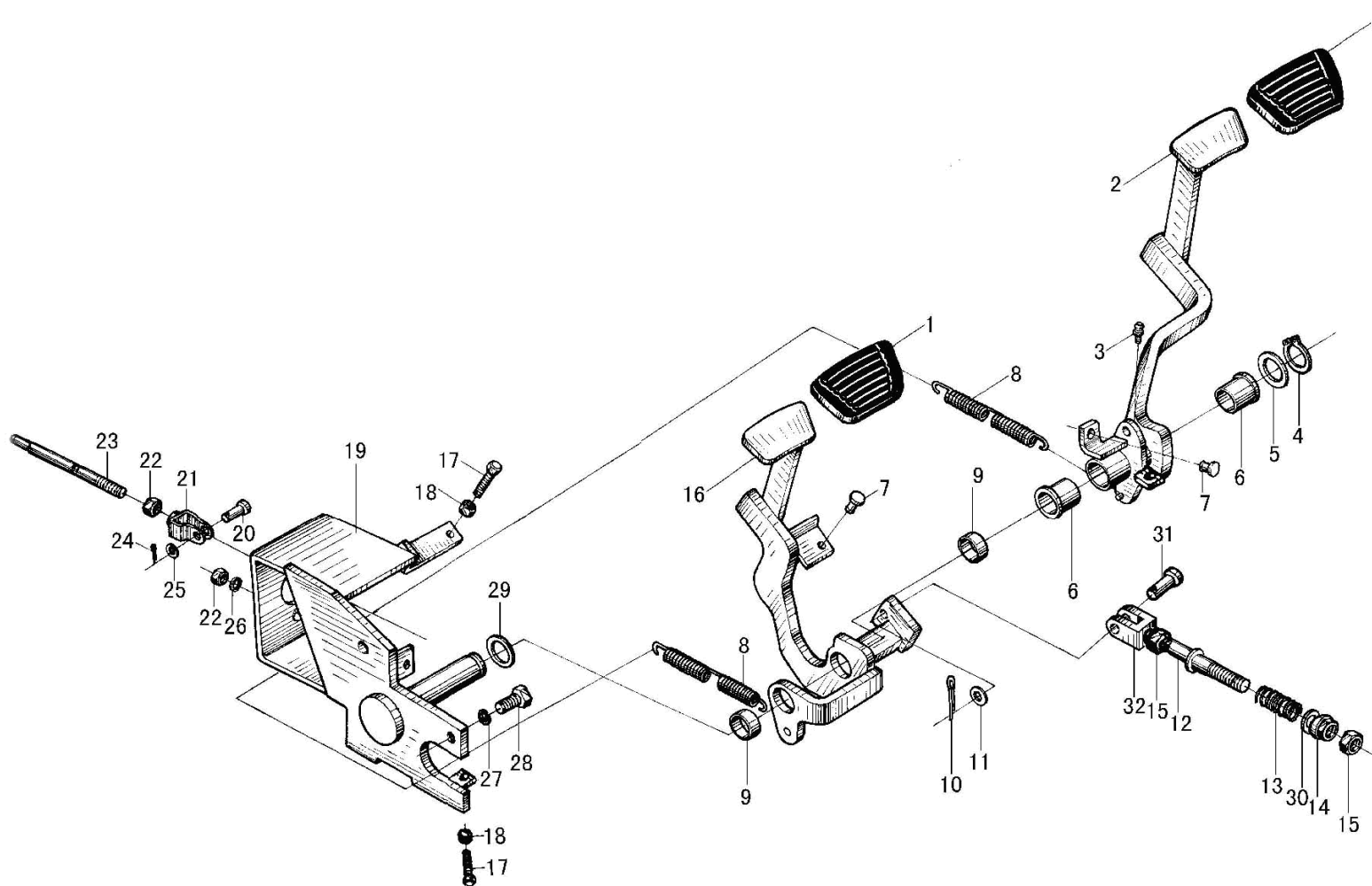
图 1 制动离合踏板总成 Fig. 1 Brake clutch pedal assy
