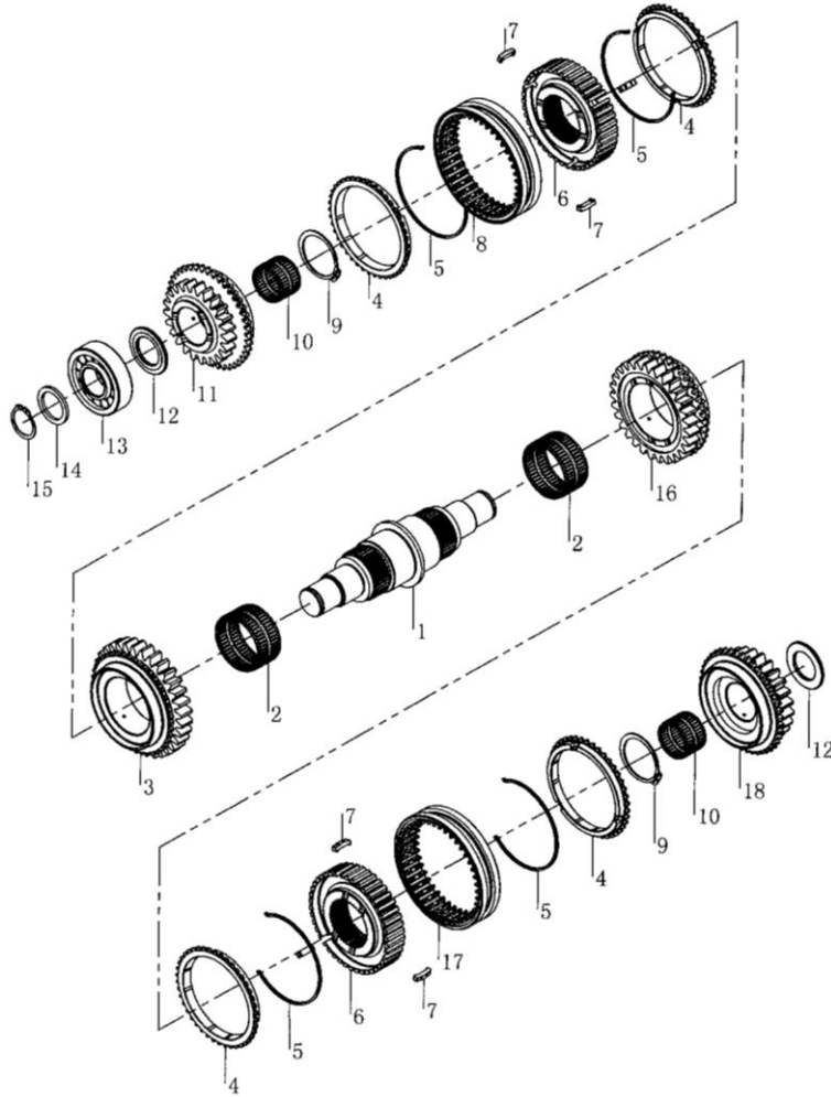
图 17-a 主轴组件 (绍兴) Fig.17-a Spindle assy (ShaoXin)
