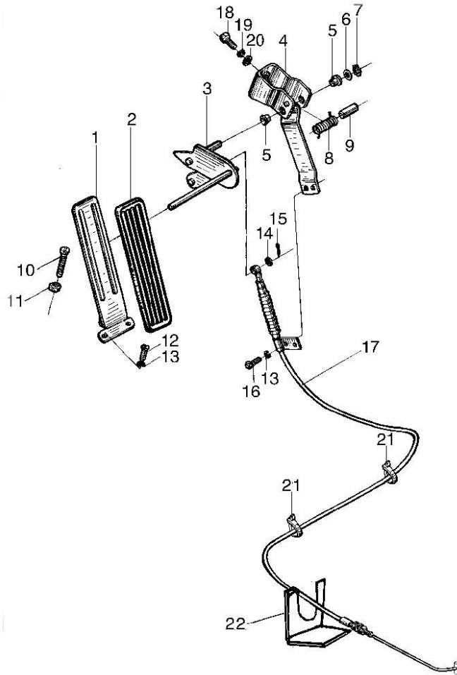
图 11 油门操纵总成 Fig. 11 Throttle control assy
