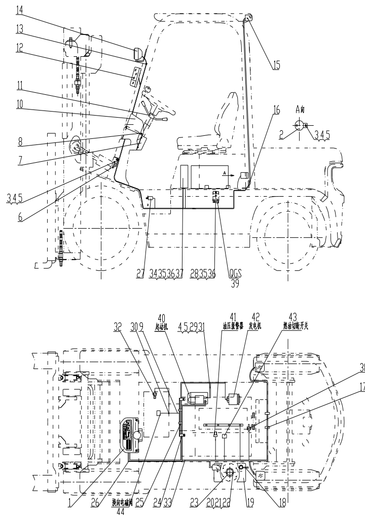
图 11 电气系统 Fig.11 Electrical system
