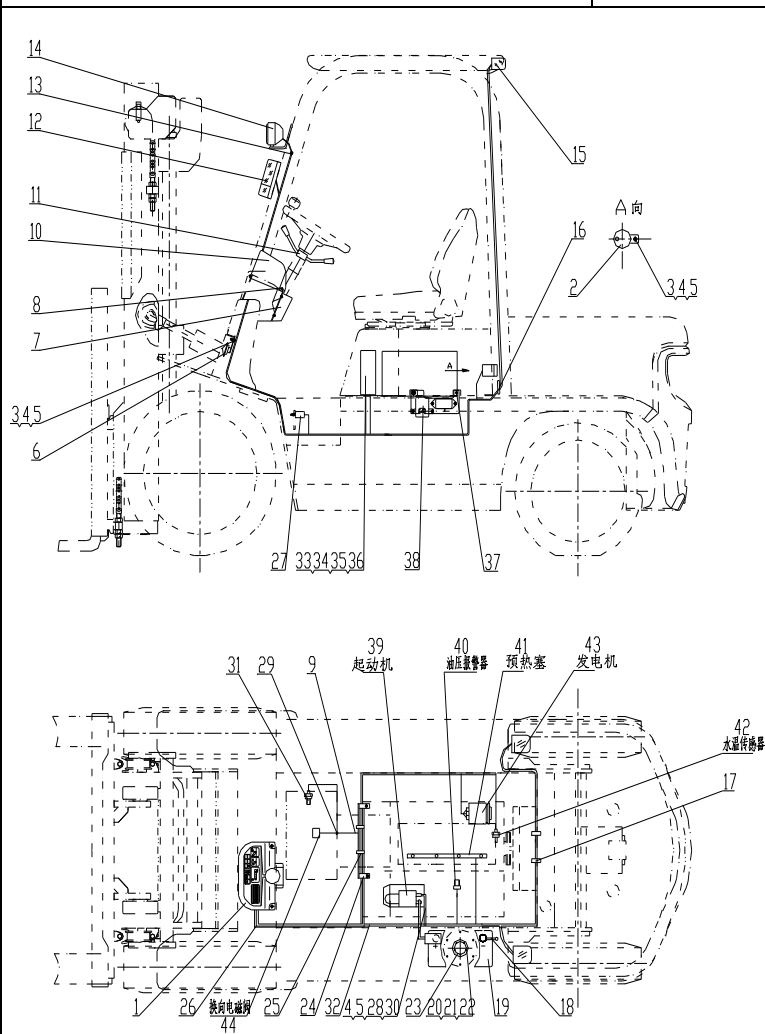
图 2-2 电气系统 Fig.2-2 Electrical system
