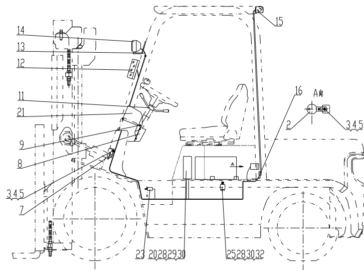
图 6-2 电气系统 Fig.6-2 Electrical system
