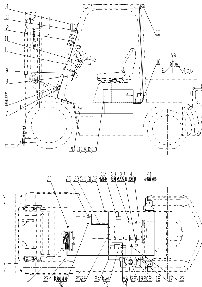
图 10-2 电气系统 Fig.10-2 Electrical system
