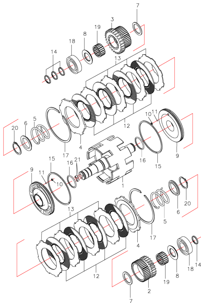
图 27 液力离合器(液力式) 中南 ZhongNan Fig.27 Hydraulic clutch(tor-con type)
