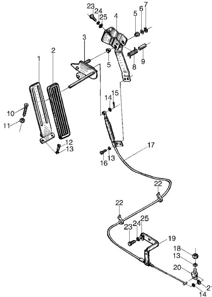
图 9 油门操纵总成 Fig. 9 Throttle control assy
