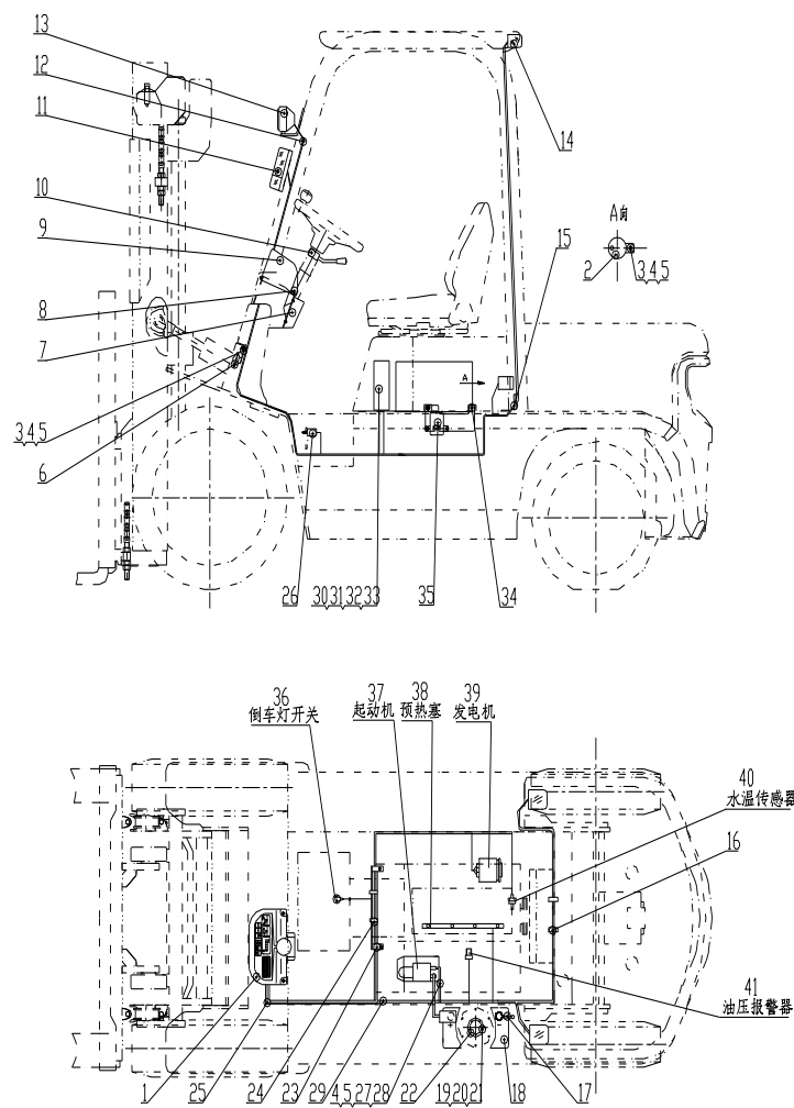
图 2-1 电气系统 Fig.2-1 Electrical system
