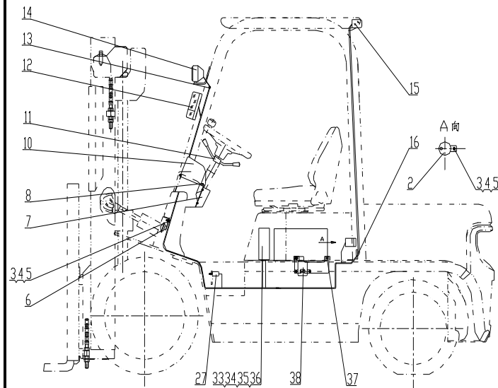
图 8 电气系统 Fig. 8 Electrical system
