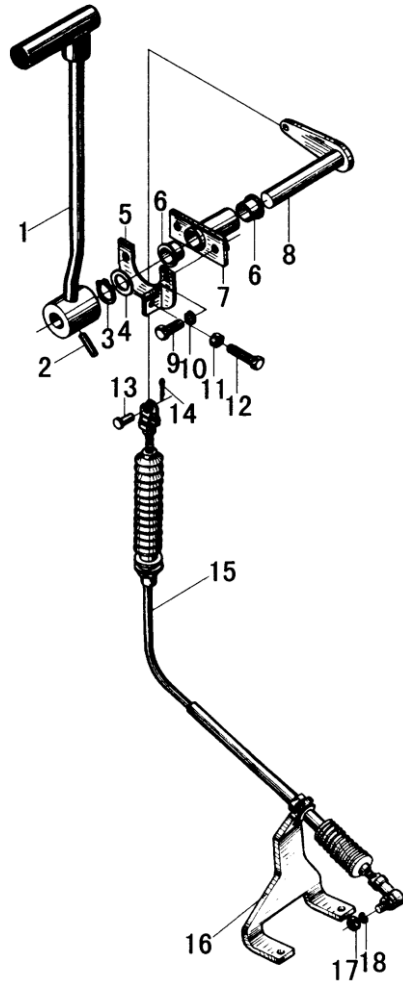
图 14 换档操纵总成 Fig. 14 Change over control assy
