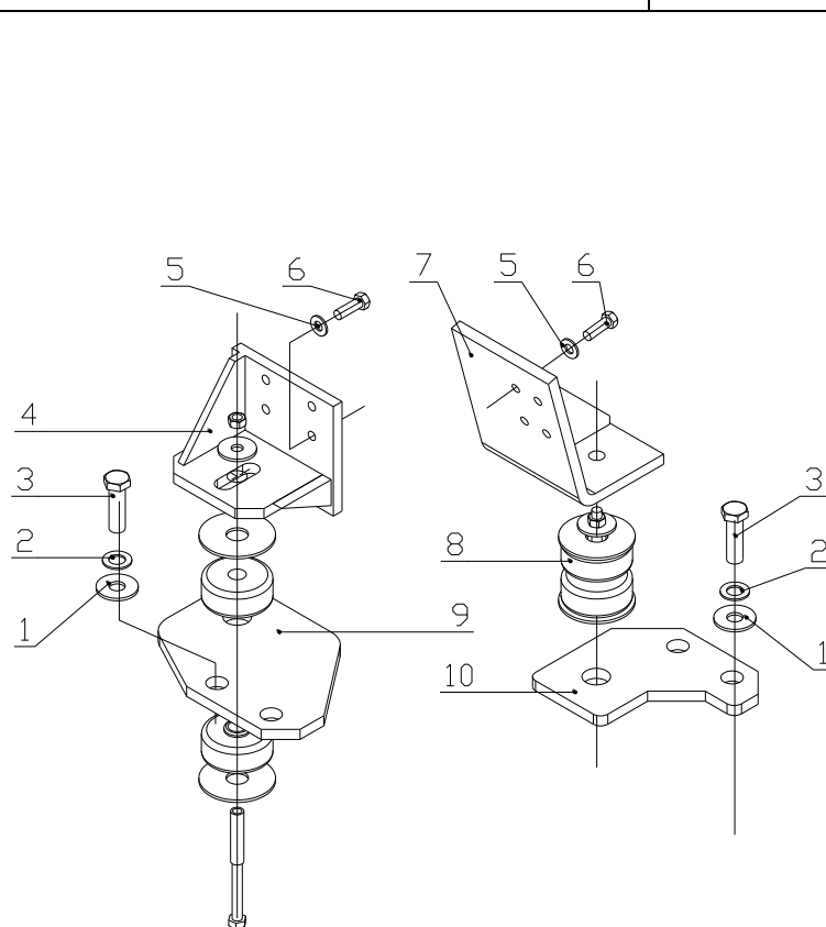
图 55 发动机安装 Fig.55 Engine mount
