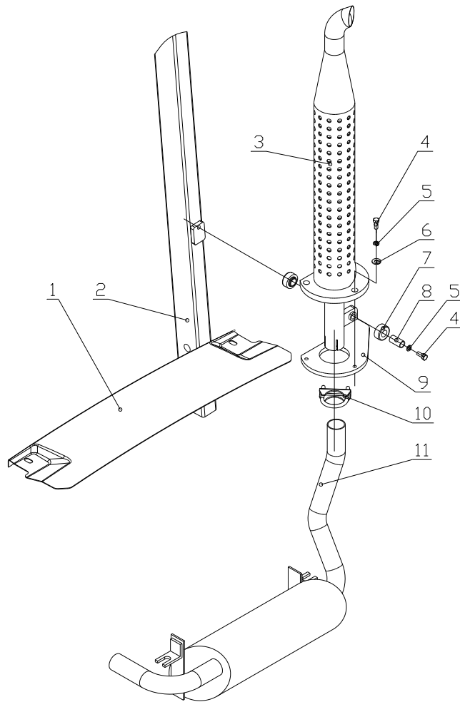
图 57 高位排气系统 Fig.57 High Exhaust system
