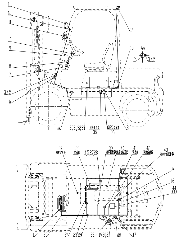
图 4-1 电气系统 Fig.4-1 Electrical system
