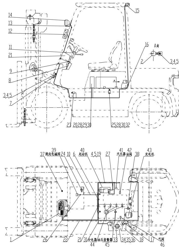
图 6-2 电气系统 Fig.6-2 Electrical system
