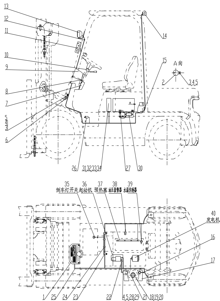
图 1-1 电气系统 Fig.1-1 Electrical system
