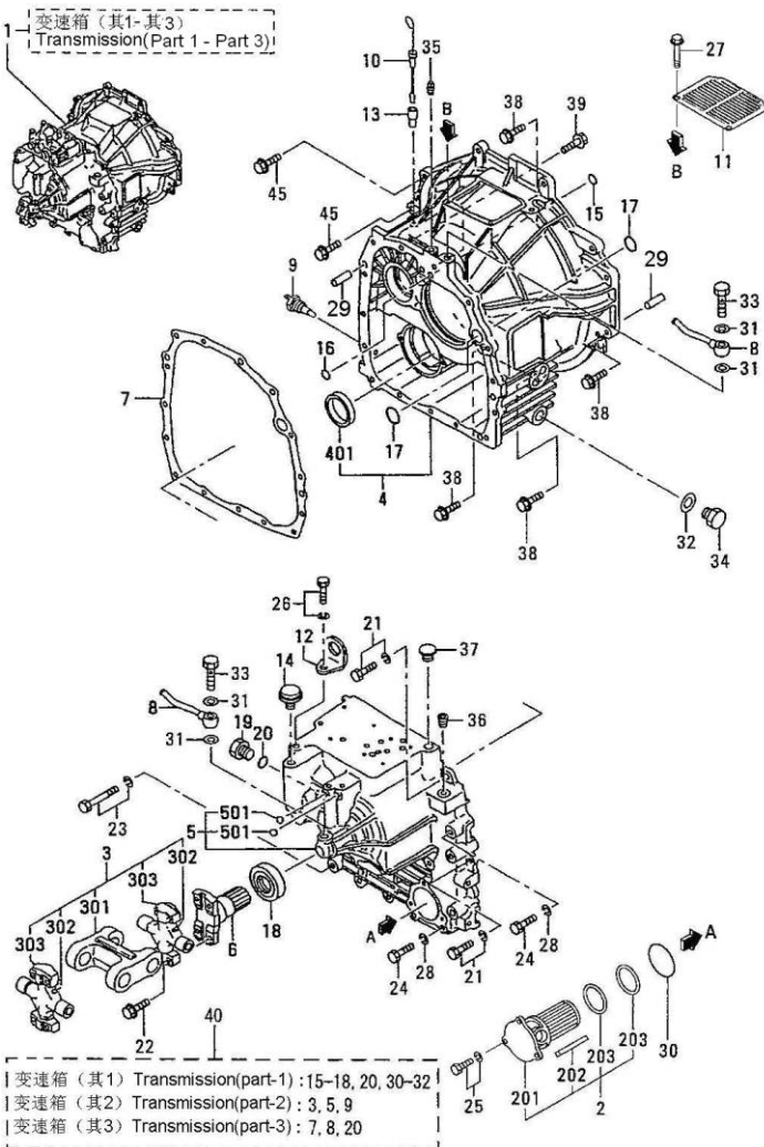
图 33 变速箱（其 1） Fig.33 Transmission (part-1)
