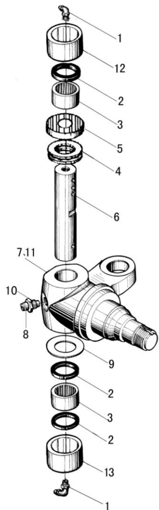
图 2 转向桥 (2) Fig. 2 Steering axle (2)
