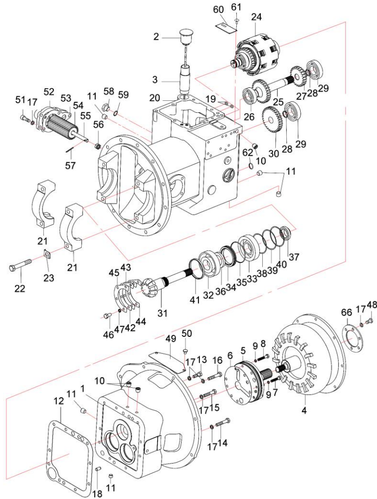
图 26 变速箱（液力式）中南 ZhongNan Fig. 26 Transmission(tor-con type)
