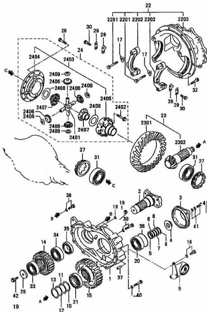
图 37 3.0-3.5t 主减速器・差速器总成 Fig.37 3.0-3.5t Reduction & Differential
