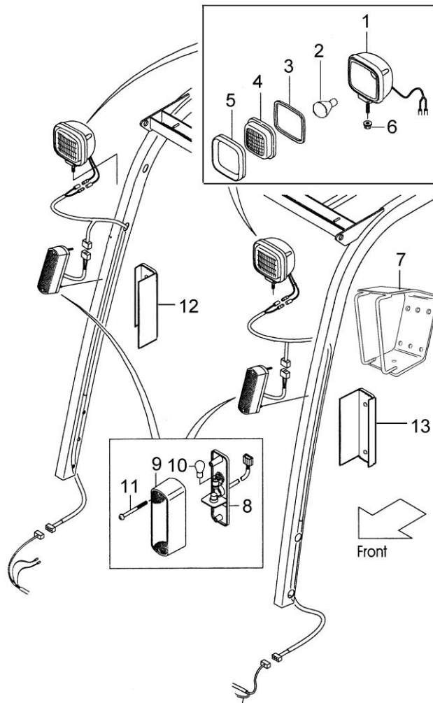
图V 前灯总成 Fig. V Front lamps assy
